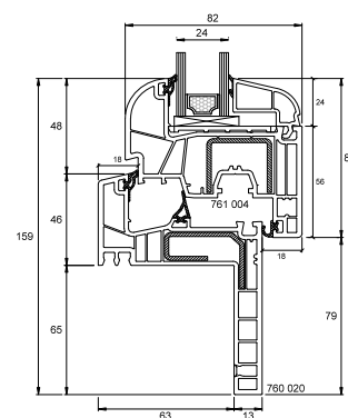
Telaio Z 65 mm
