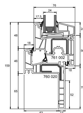
Telaio Z 65 mm
