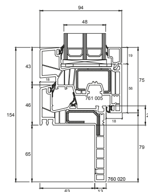
Telaio Z 65 mm
