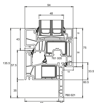
Telaio Z 35 mm
